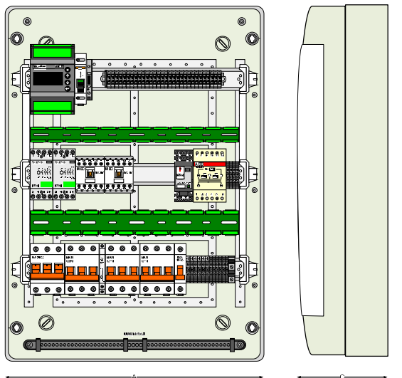
Расположение элементов внутри щита управления.
