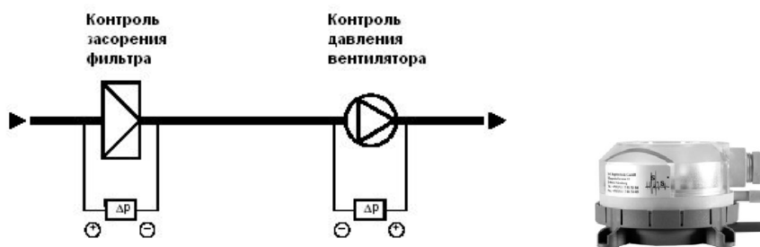
Внешний вид и примеры использования датчиков давления.
