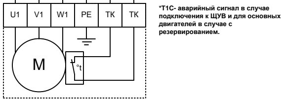
Двигатель вентилятора
