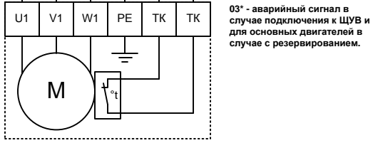
Двигатель вентилятора
