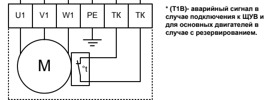
Двигатель вентилятора
