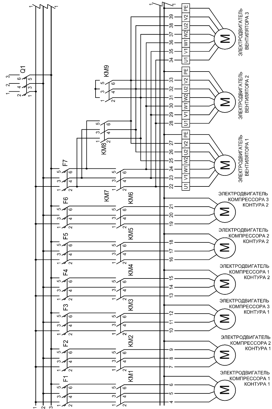
Принципиальная электросхема агрегатов 177D и 206D (лист 1)
