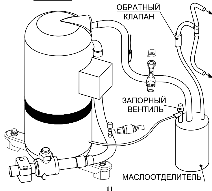
Рисунок 3.5.3. Схема монтажа опции маслоотделителя для модели 071D
