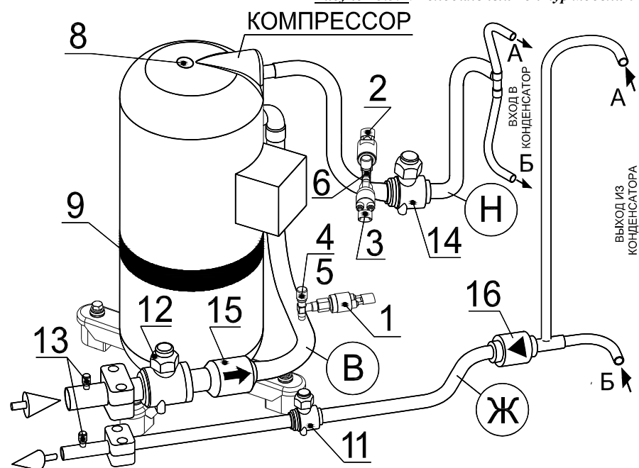
Рисунок 3.5.3. Схема монтажа опции маслоотделителя для модели 071D
