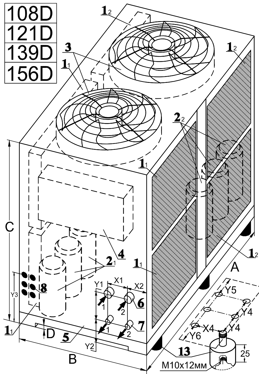
Рисунок 1.1. Компоновка и основные размеры агрегатов
