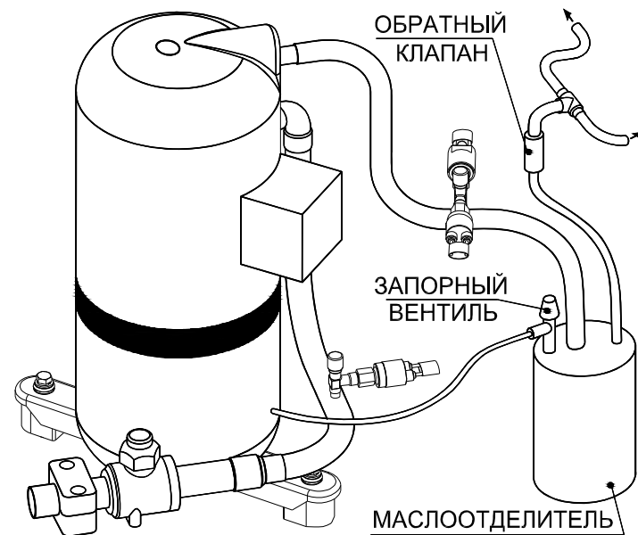
Рисунок 3.5.3. Схема монтажа опции маслоотделителя для моделей 024÷035
