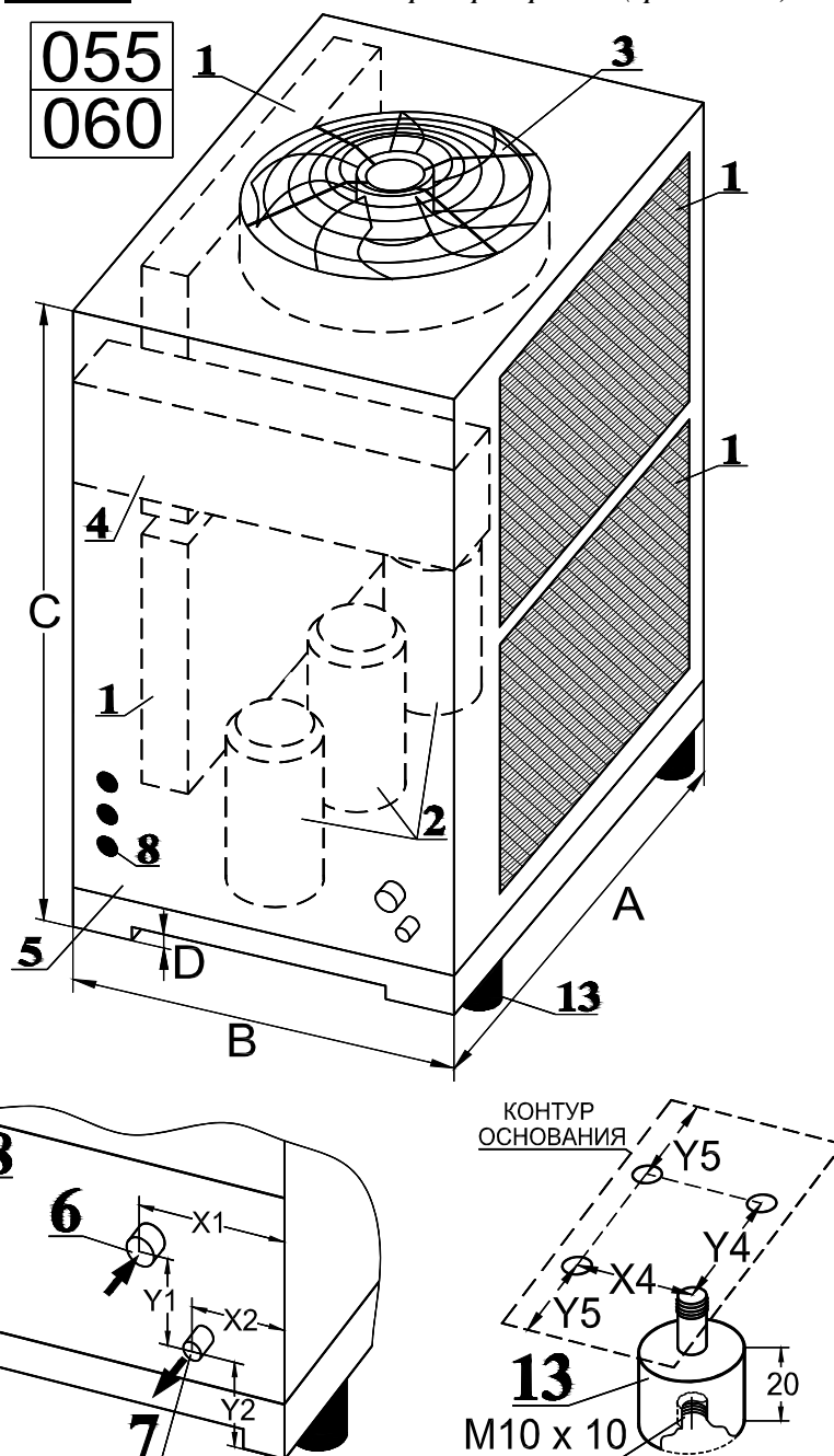
Рисунок 1.1. Компоновка и основные размеры агрегатов (продолжение)
